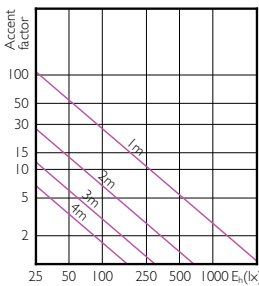
MASTER LEDspot PAR 60W E27 827 25D
