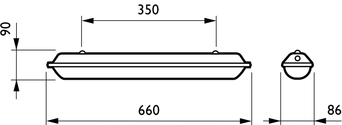
Méretezett rajza
