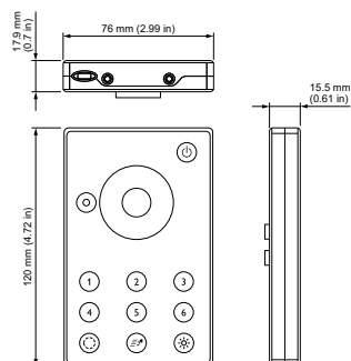
Vaya controls VAYACT
