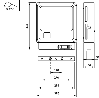
MINI 300 LED gen2 BBP/BCS/BVS400
