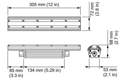
BCS419 10x60-3000 L305
