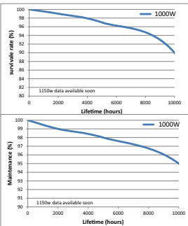
Life Expectancy Diagram - HPS AGRO Plus 1000W DE EL
