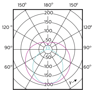
(cd/1000lm) 0° — 0-180° — 90-270°
