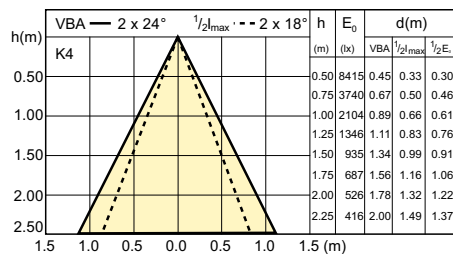
LDBE_CDM-Rm_20W_40D_0003-Beam diagram
