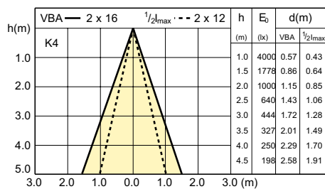
LD BE_HALUACN_50W_24D-Beam diagram
