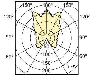
(cd/1000lm) 0°
