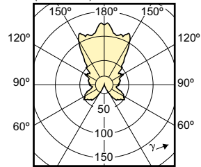
(cd/1000lm) 0°
