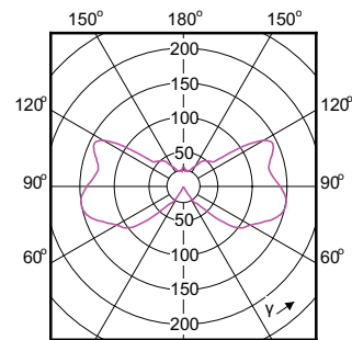
(cd/1000lm) 0°
