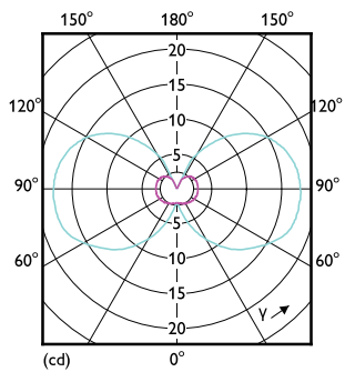
(cd) 0-180° 90-270°
