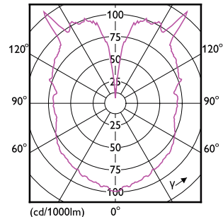
(cd/1000lm) 0°
