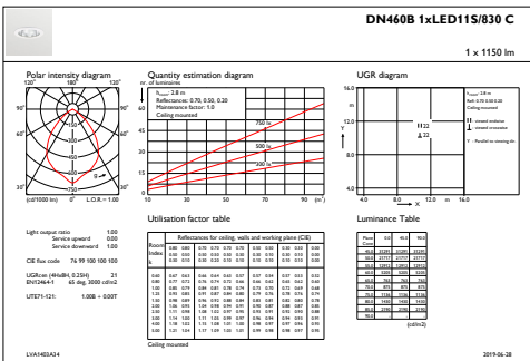
IFGU1_DN460B1xLED11S830C
