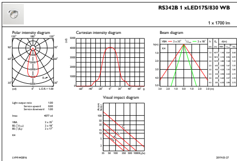
IFAS1_RS342B1xLED17S830WB
