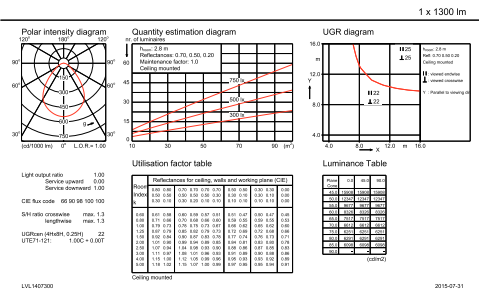
DN570B PSED-E 1xLED12S/830 WR
