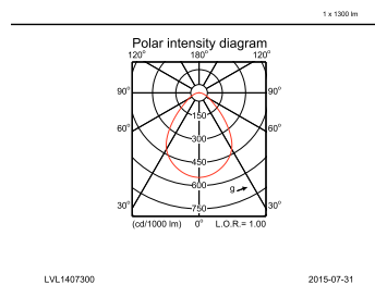
DN570B PSED-E 1xLED12S/830 WR
