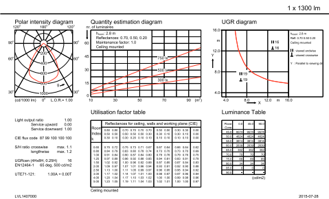
DN571B PSED-E 1xLED12S/840 F
