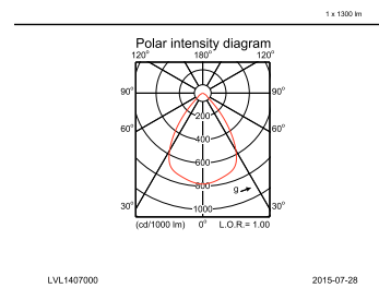
DN571B PSED-E 1xLED12S/840 F
