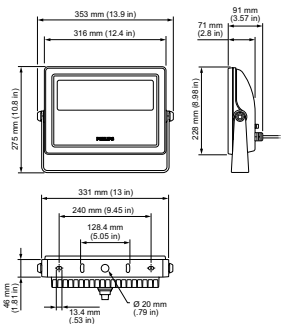
BCP435 4000 120-277 40 UL
