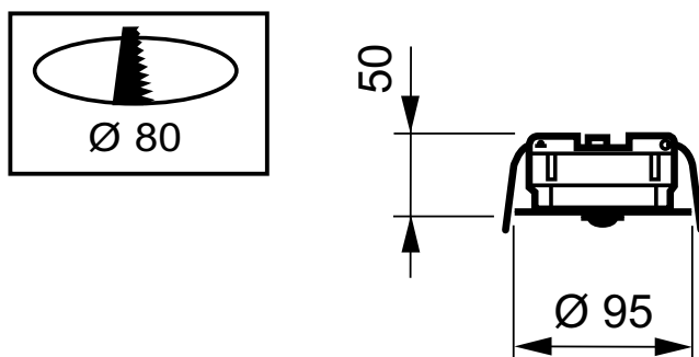
LRM1085/00 SENSOR MOV DET ST IR CH
