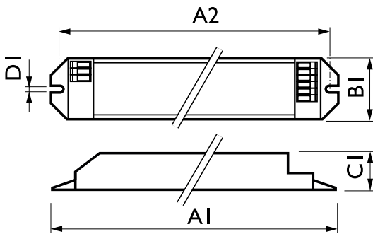
EB-C 121 TL5 220-240V 50/60Hz
