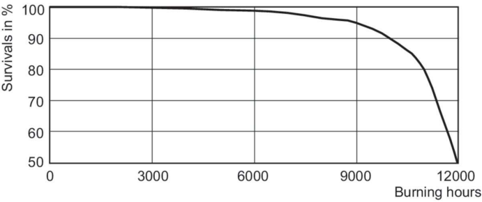
Life Expectancy Diagram - MASTERC CDM-TM MINI 35W/930 PGJ5 KIT/12
