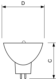
13528 15W GZ4 6V
