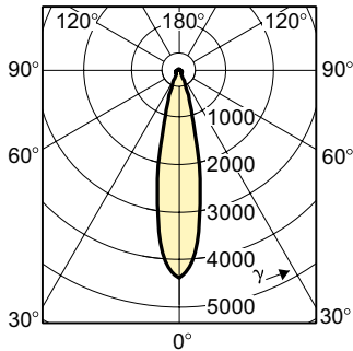
Halogen Dichroic 50W 24D
