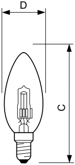
HalClass 18W E14 230V B35 CL
