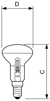
HalClass 28W E14 230V R39 45D FR
