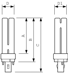
PL-C 13W/827/2P
