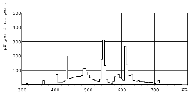
Lichtfarbe TL-D de Luxe /950
