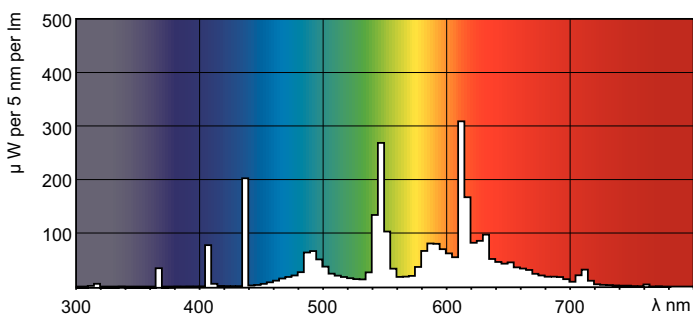
Barwa Światła TL-D de Luxe /930
