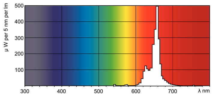
Barwa Światła TL-D /150
