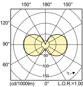
Light Distribution Diagram - MASTERC CDM-Tm Mini 20W/830 PGJ5 1CT/12
