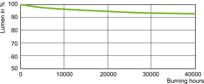
Lumen Maintenance Diagram - MST SON APIA Plus Xtra 400W E40 1SL/12
