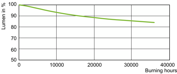
Lumen Maintenance Diagram - MASTER SON PIA Plus 400W/220 E40 1SL/12
