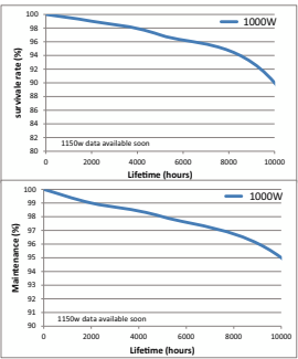
Life Expectancy Diagram - HPS AGRO Plus 1000W DE EL 1CT/12
