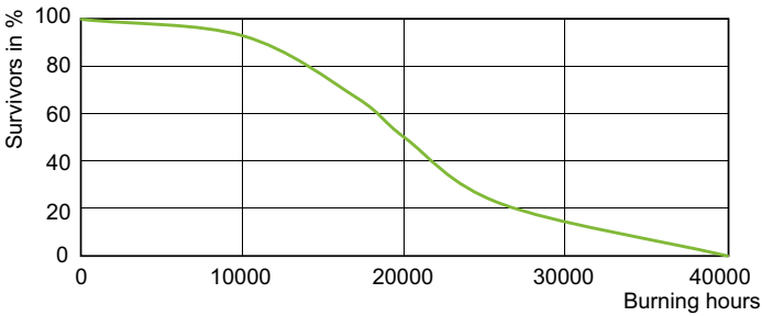
Life Expectancy Diagram - CDM145/C/U/O/4K/ED28 EA Allstart
