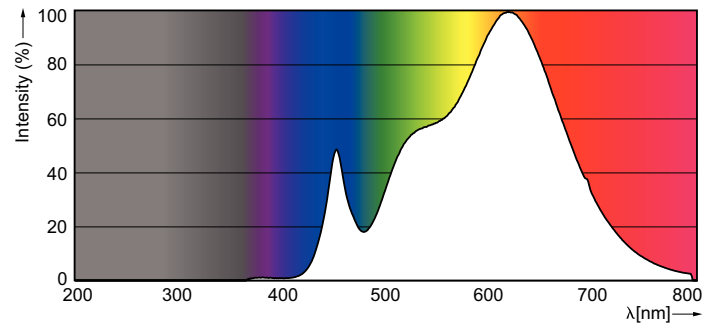
11-50W AR111 /930
