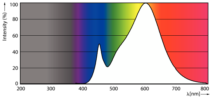
Spectral Power Distribution Colour - BC3 G9 Capsule AMB 3000 ND 120V
