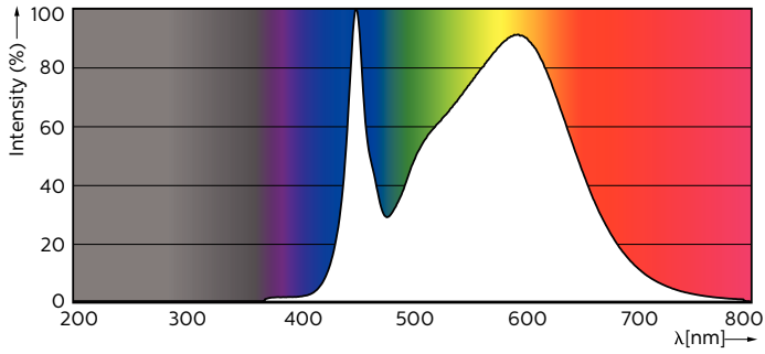
LEDtube 1500mm HO 20W840 T8
