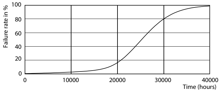
LEDspot 50W GU10 830 35D
