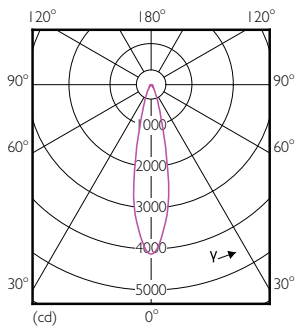
12-90W E26 PAR38 25D 840 4000K
