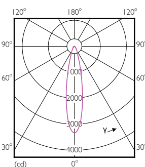
10-75W E26 PAR30L 25D 827 2700K
