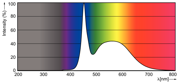
MAS LEDtube EM 14W G13 765 T8 THD
