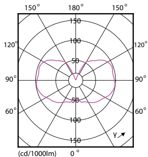
LEDbulb 14W E27 820 CL A60
