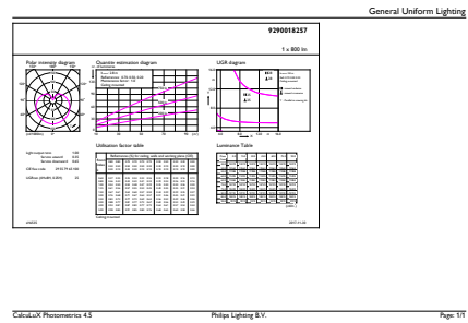
60W E26 A19 FR 250D 927 2700K
