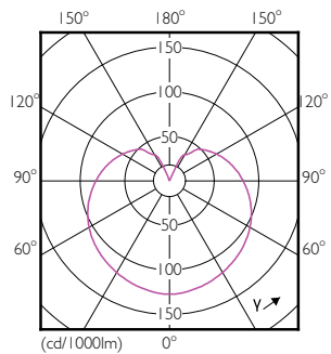
60W E26 A19 FR 250D 927 2700K
