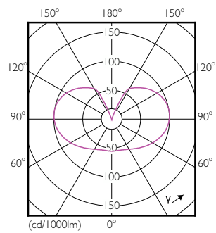
Light Distribution Diagram - 5G25/PER/827/FR/G/DIM 6/1CT
