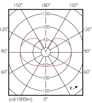
Light Distribution Diagram - 5G25/PER/827/FR/G/DIM 6/1CT
