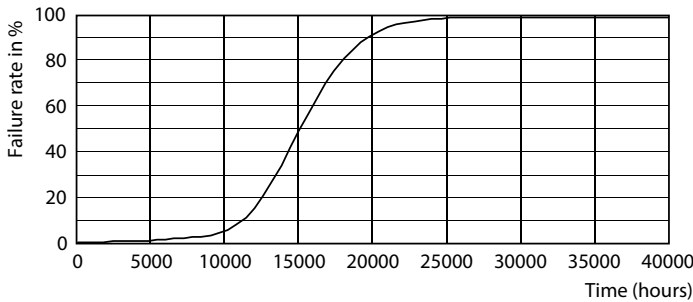
Life Expectancy Diagram - 5G25/PER/827/FR/G/DIM 6/1CT
