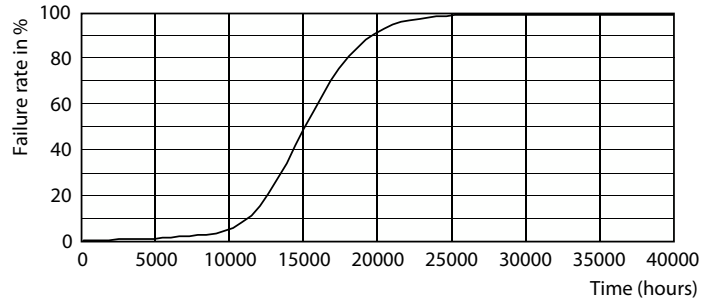
Life Expectancy Diagram - 4.5BA11/PER/850/CL/G/E12/DIM 6/1CT
