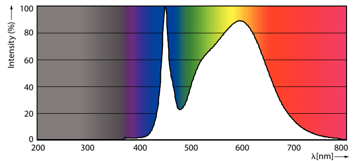
14W G13
