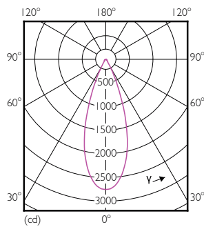
LEDspot PAR38 E26 927 40°
