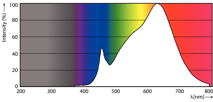
LEDspot PAR20 E26 3000K
