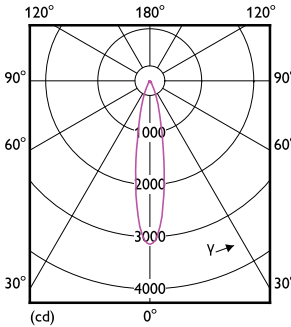
LEDspot PAR20 E26 3000K 25D
